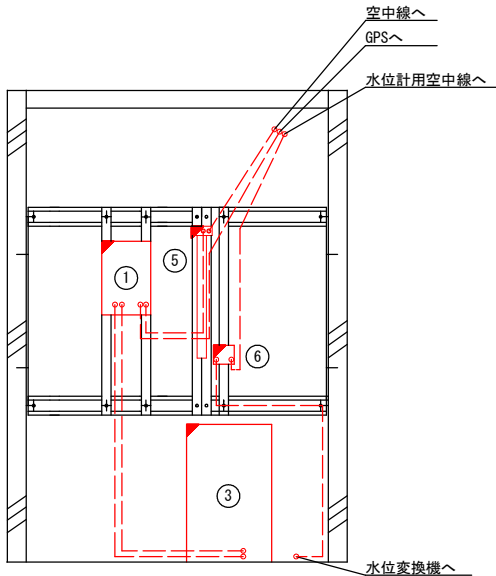
立面図（内視）（“A”より望む）
