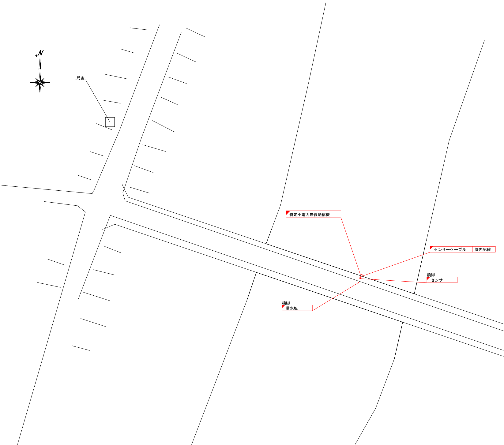
敷地平面図 S=1/250
