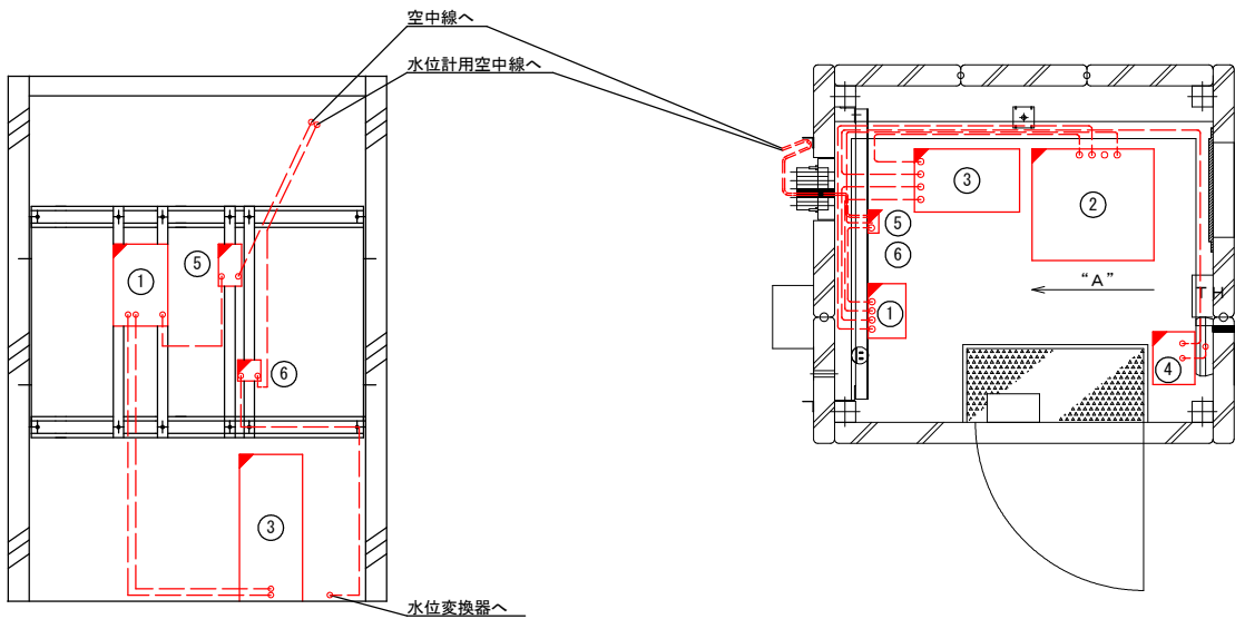
立面図（内視）（“A”より望む）
